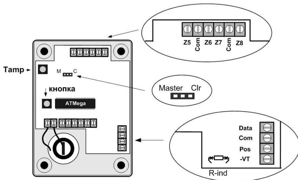
Рис. 3 Вид сзади
