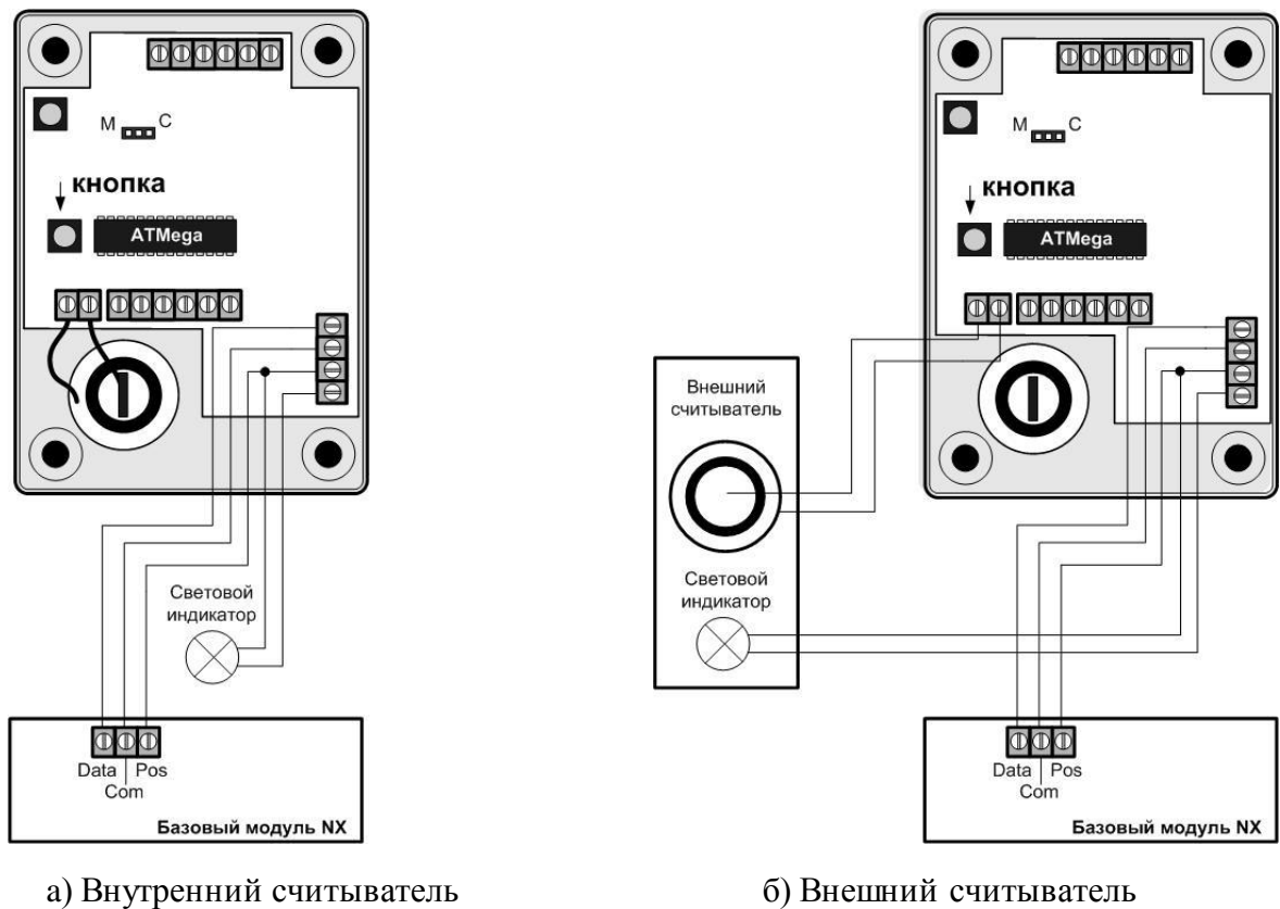
Рис.4 Подключение к системной трех проводной шине
