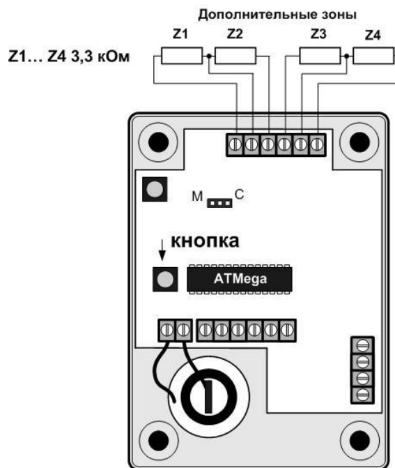
Рис.5 Схема подключения дополнительных зон
